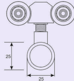
SLIDING DOOR ROLLER
